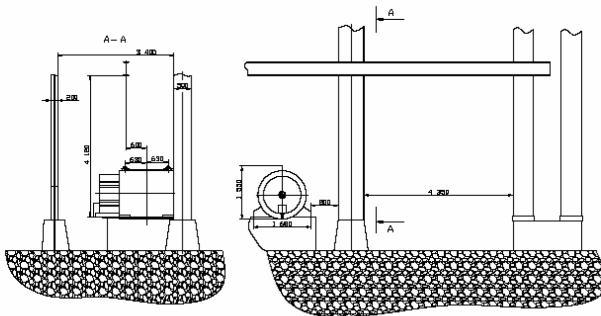
Схема на разположение на двигател за МВ 1Б
