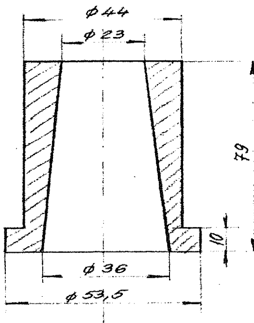
Дюза за хидроциклон
