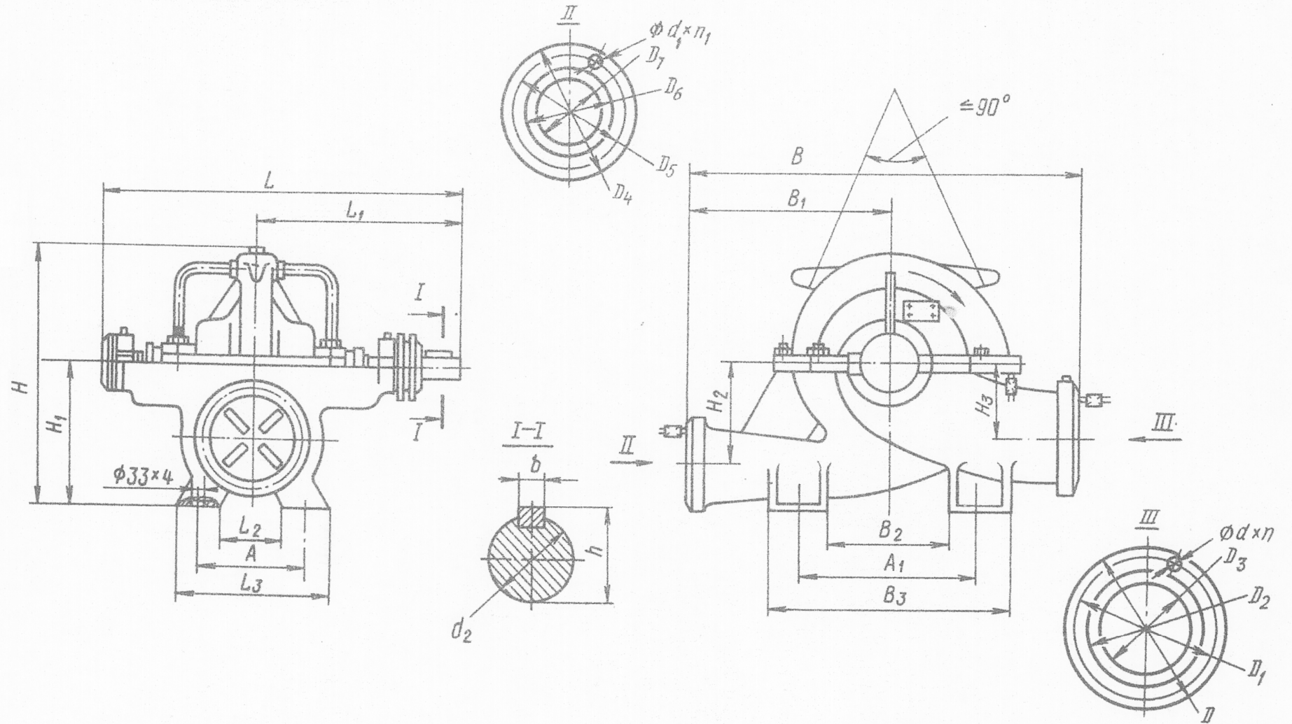
Приложение №4- Габаритни и присъединителни размери на помпата
